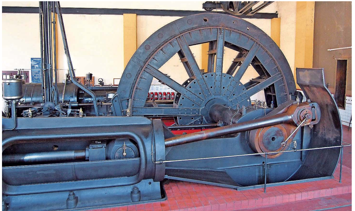
Im Erlebnisbergwerk Velsen kann die älteste Dampfförder-Maschine des Saarlandes besichtigt werden. Foto: Reinhardt
